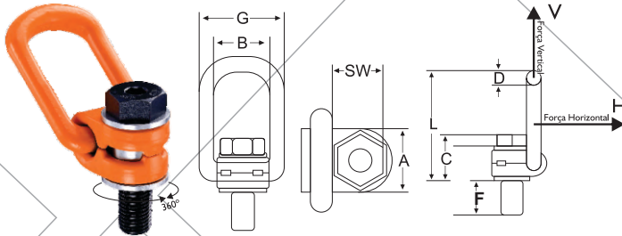
Olhal Aparafusável Giratório - OGL
