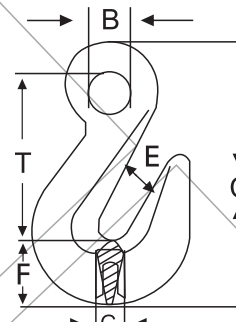
Gancho Olhal Encurtador - Aço alloy GRAU 10
