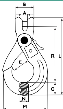
Gancho clévis automático - Aço alloy GRAU 10
