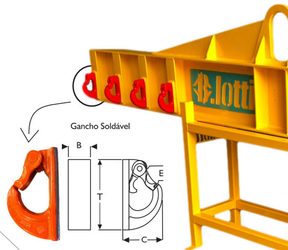
Gancho Soldável - Aço alloy GRAU 8
