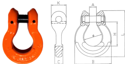
Conector Omega - Aço alloy GRAU 8
