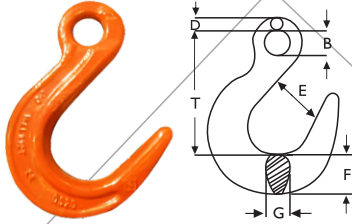
Gancho Olhal de Fundição - Aço alloy GRAU 8
