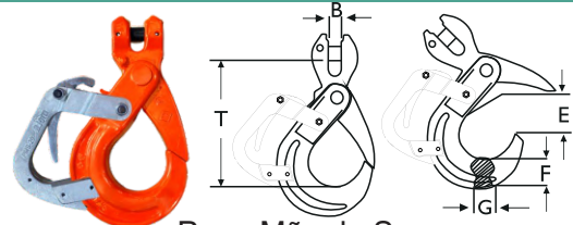
Pega Mão de Segurança Gancho Clévis Automático - Aço alloy GRAU 8
