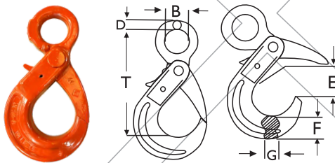
Gancho Olhal Automático - Aço alloy GRAU 8
