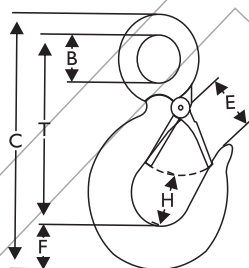
Gancho Olhal com trava de segurança
