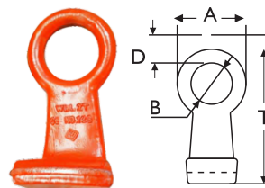
Gancho Olhal para Tambor - Aço alloy GRAU 8
