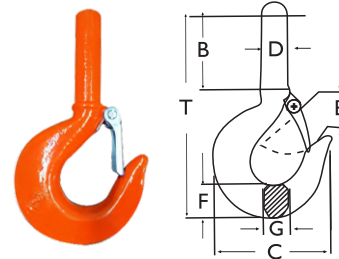
Gancho Haste - Aço carbono - com trava de segurança
