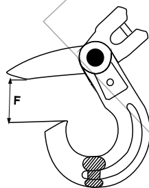
Gancho clévis automático - Aço alloy GRAU 10
