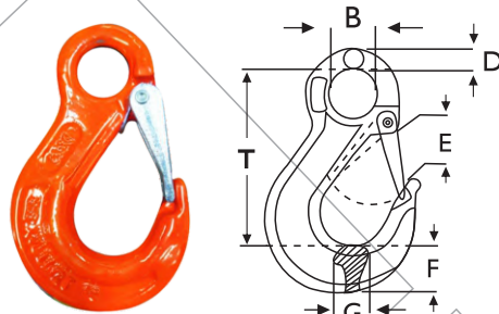
Gancho Olhal - Aço alloy GRAU 8
