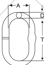
Elo de Sustentação - Aço alloy GRAU 8
