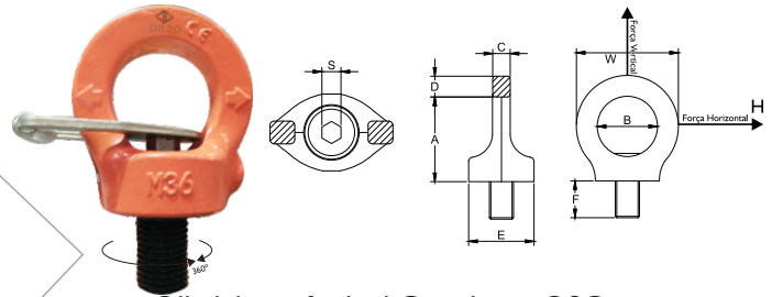
Olhal Aparafusável Giratório - OSG
