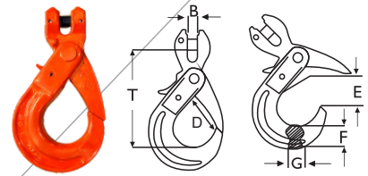
Gancho Clévis Automático - Aço alloy GRAU 8
