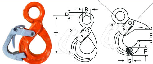
Pega Mão de Segurança Gancho Olhal Automático - Aço alloy GRAU 8
