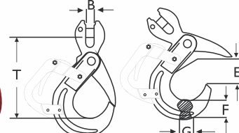
Pega Mão de Segurança Gancho Clévis Automático - Aço alloy GRAU 8
