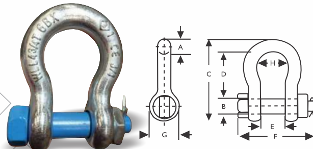
Manilha Âncora - Porca e Cupilha
