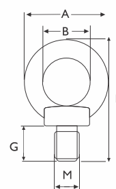
Olhal Aparafusável Fixo - Grau 8 Parafuso Olhal (OPA)
