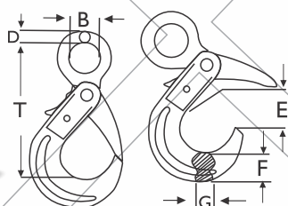
Gancho Olhal Automático - Aço alloy GRAU 8
